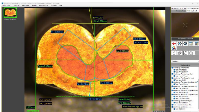
Vermessenes Schliffbild mit X-Scan
